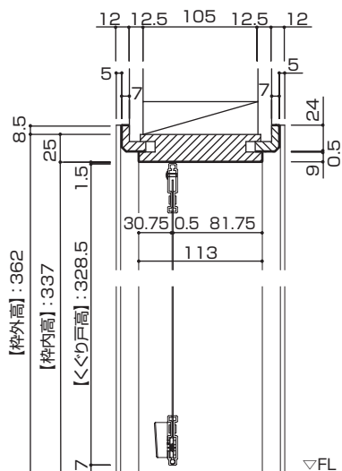
縦断面図
