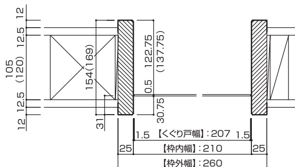
横断面図
